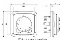
Přístroj s krytem a námočkem
