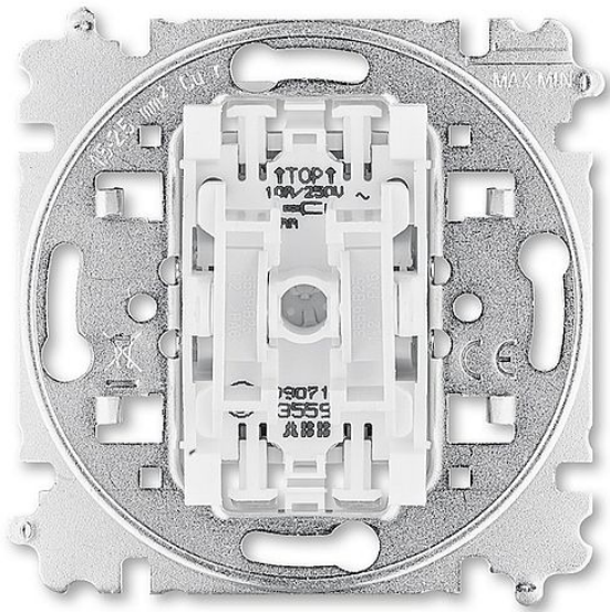
Spínač / ovládač žaluziový kolébkový (s mechanickým blokováním)
